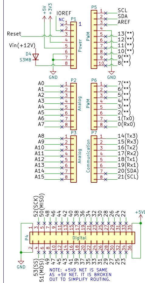
ARDUINO MEGA REV 3
